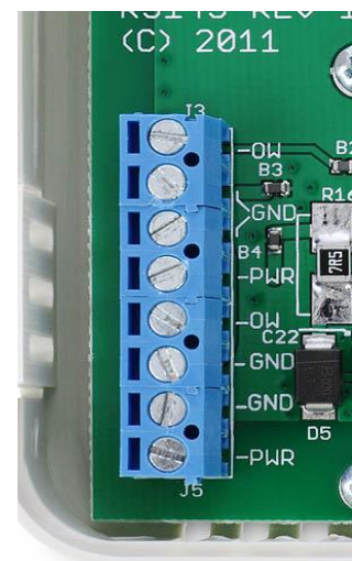
Abb. Sensorklemmen
